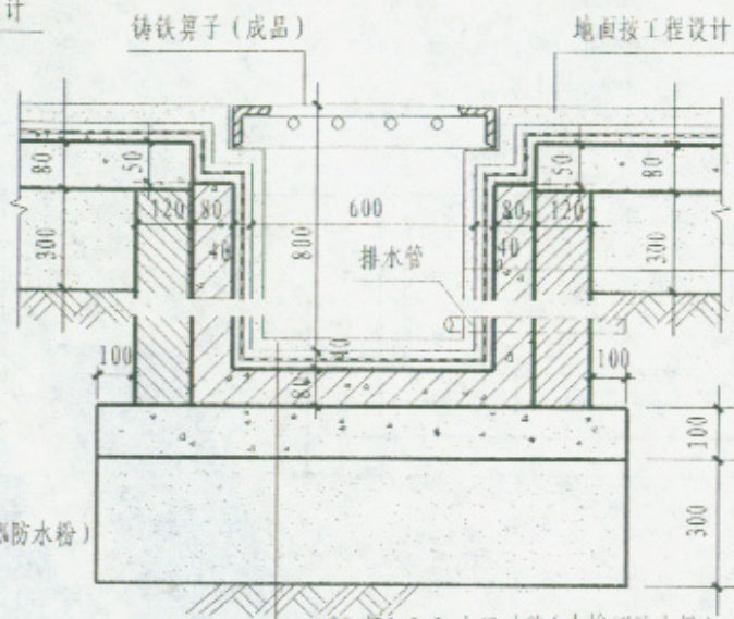
A-A (用于自重性湿陷性黄土场地) 20厚1:2.5水泥砂浆 防水层 (材料由设计人定) 20厚1:2.5水泥砂浆 80厚C25混凝土 (内配钢筋 \Phi 8 中距200双向) 120厚烧结砖砌体
