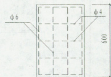
A 沟盖板
