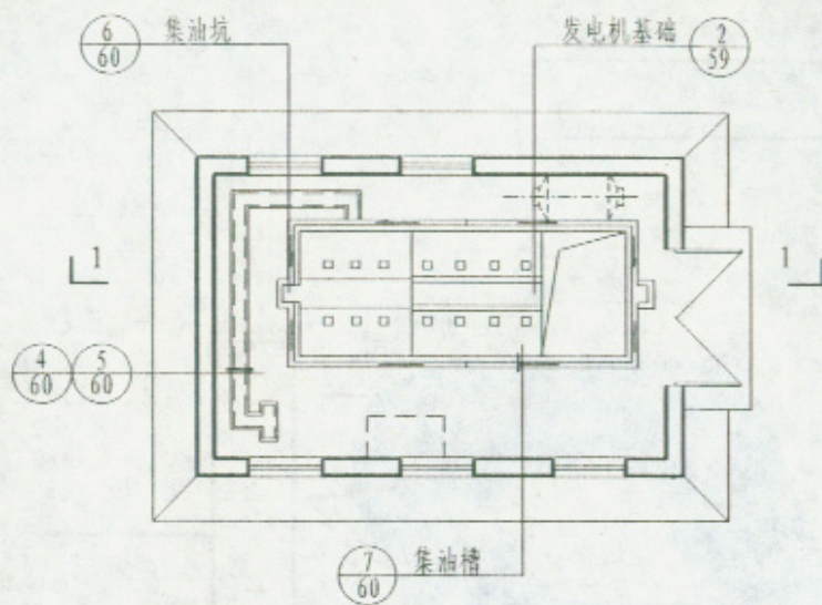
平面示例
