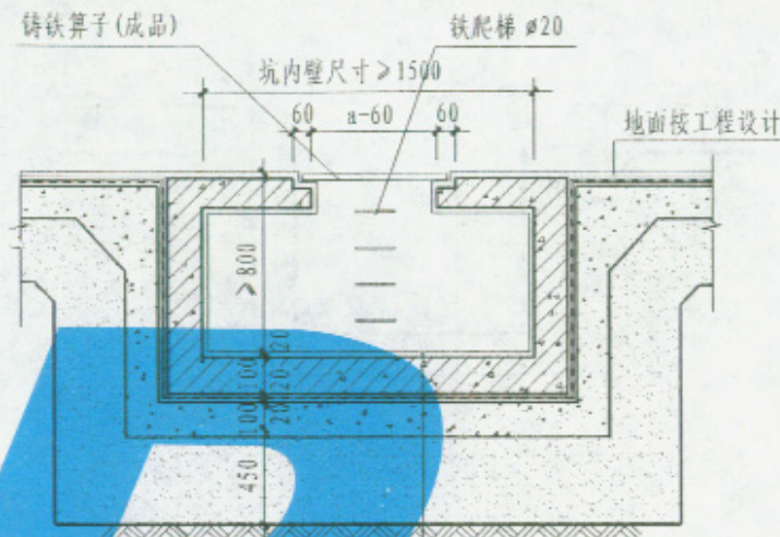
② 集水坑 (用于湿陷性黄土场地)
