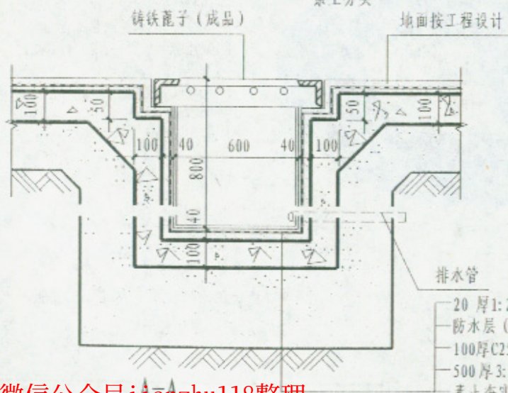
A-A (用于非自重湿陷性黄土场地) 20厚1:2.5水泥砂浆 (内掺5%防水粉) 防水层 (材料由设计人定) 100厚C25混凝土 500厚3:7灰土 素土夯实
