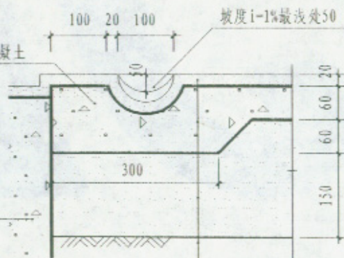
7 集油槽
