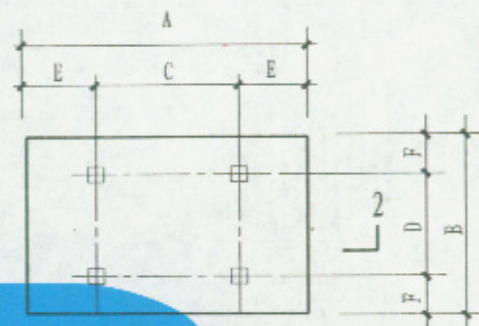
水泵基础平面
