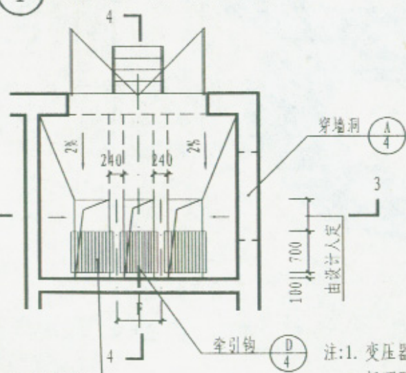
① 变压器室平面示例(墙式)
