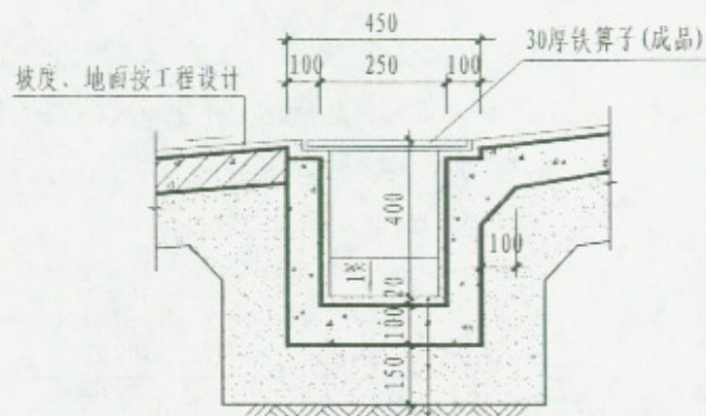
① 截水沟
