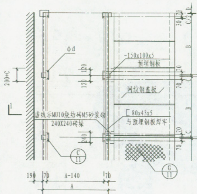
平面 1 (砖砌沟壁) 2 (混凝土沟壁)
