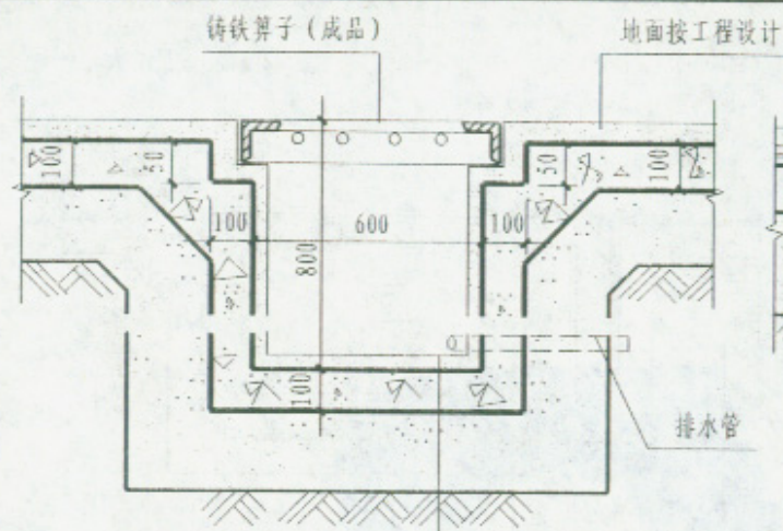
A-A (用于非自重湿陷性黄土场地) 20厚1:2.5水泥砂浆 (内掺5%防水粉) 100厚C25混凝土 150厚3:7灰土 素土夯实
