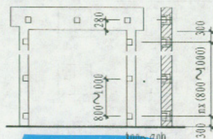
立面图
