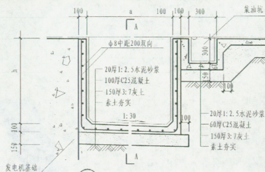
1 滑油箱坑及集油坑剖面
