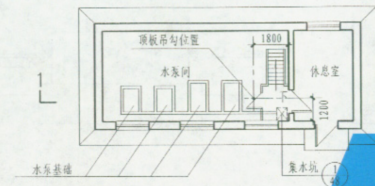
平面示例
