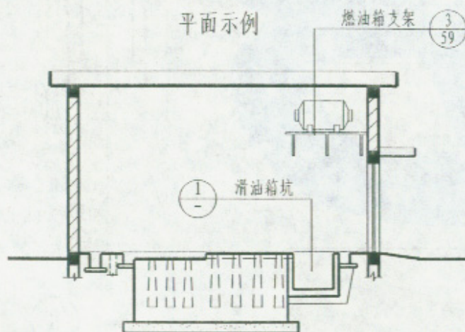
1-1 剖面
