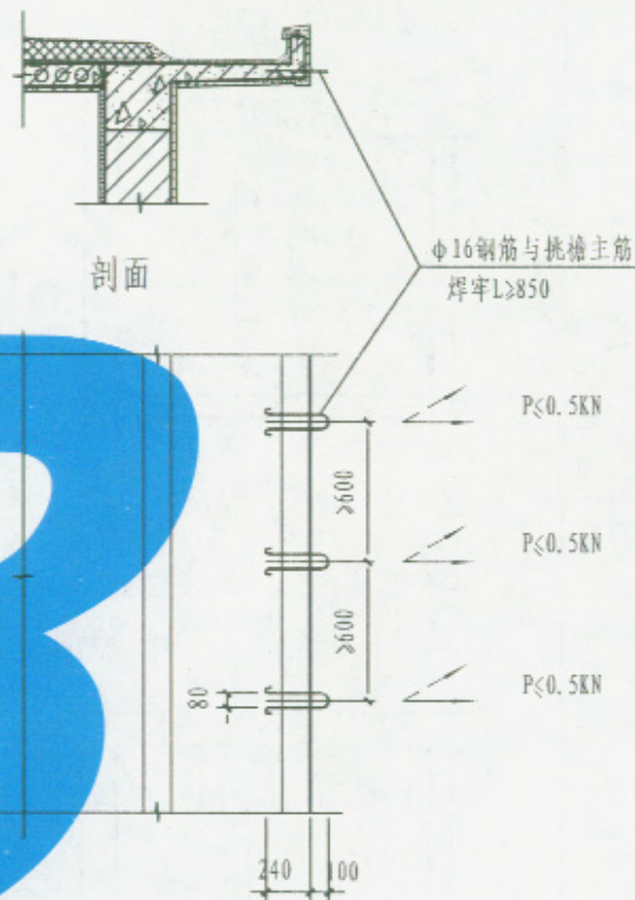
挑檐平面
