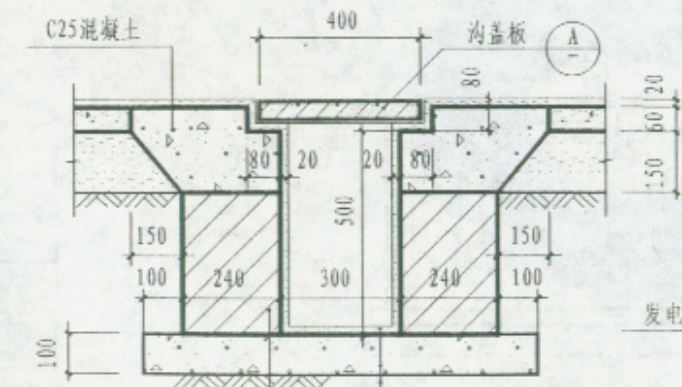
4 混凝土电缆沟
