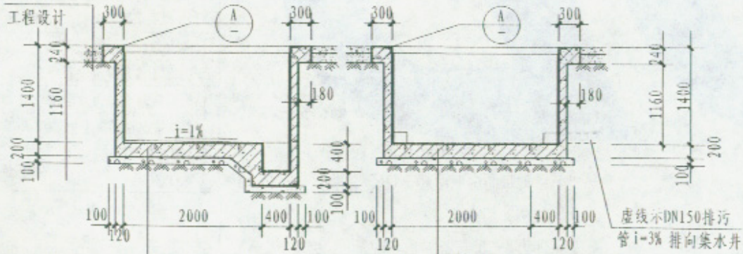
1-1 剖面
