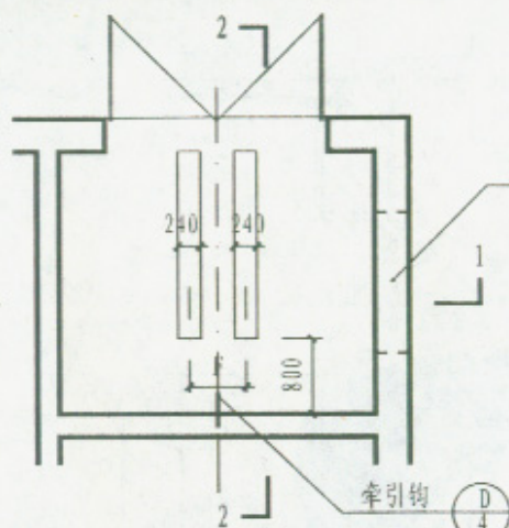
① 变压器室平面示例(墙式)
